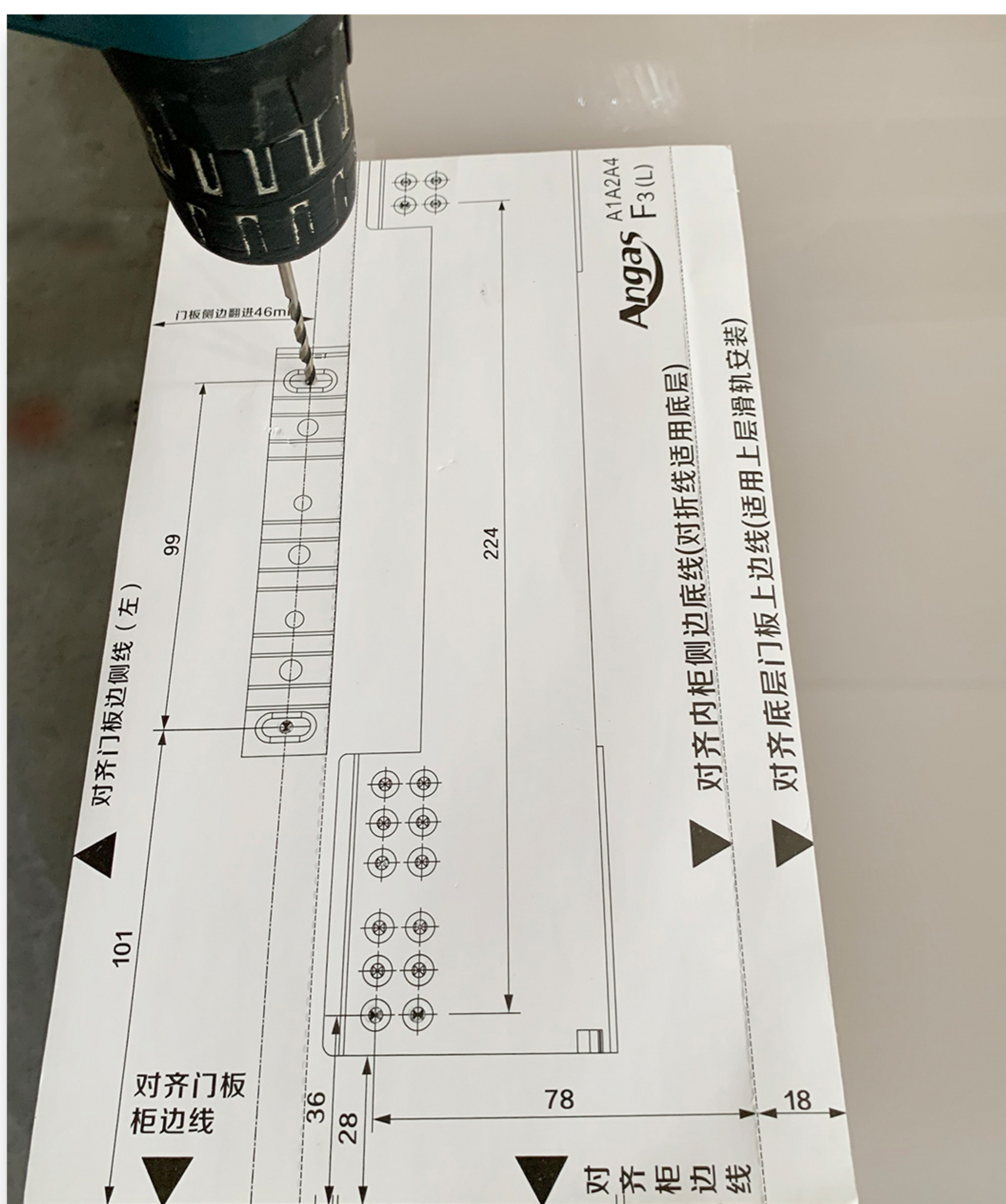
门板预钻孔（左右）
